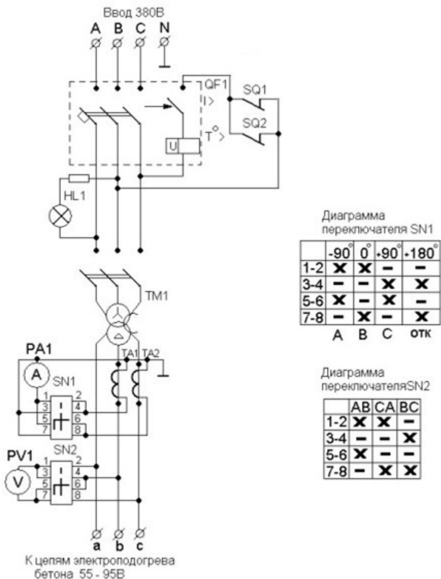
Схема электрическая принципиальная КТПТО - 80
